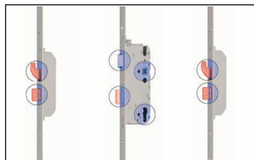
Secury Fünffach-Riegelfallenschloss (mit 2 Schwenkriegel)
