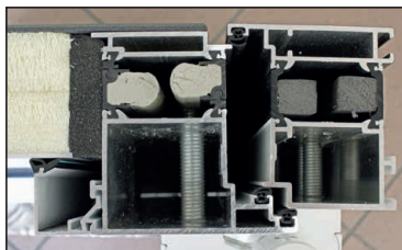
Schüco System ADS 75 Typ 75 / 85 mit aufschlagendem Flügel (3 Dichtungen)
