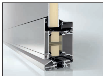
Doppelte Schwellendichtung mit gedämmter Alu-Bodenschiene EV1
